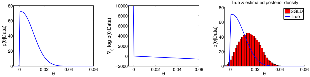
(a) Posterior density
